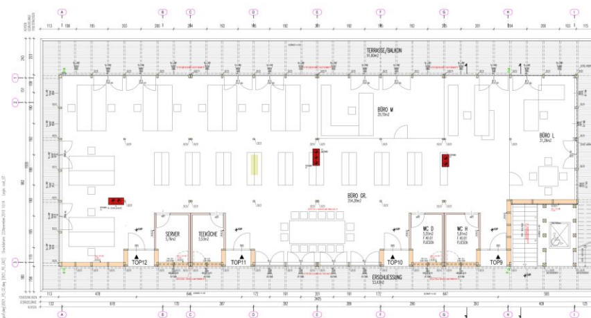
GRUNDRISS 2.OG +5,90 1:100
